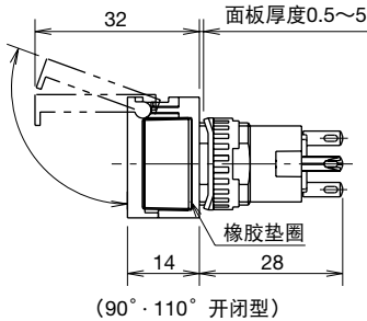
(90°·110° 开闭型)
