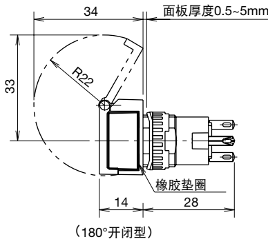
(180°开闭型)
