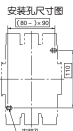
安装孔尺寸图
