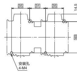
安装孔尺寸图
