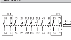
触头结构
