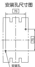
安装孔尺寸图
