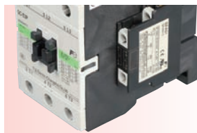
辅助触点单元（侧装） (型号: SZ-AS □)
