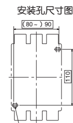
安装孔尺寸图
