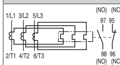
接线图
