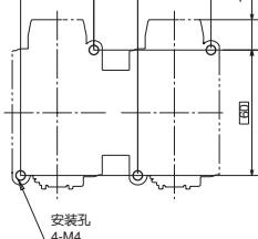
安装孔尺寸图
