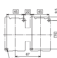
安装孔尺寸图
