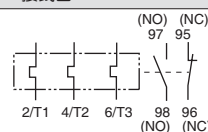
接线图
