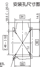
安装孔尺寸图
