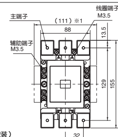
安装孔尺寸图
