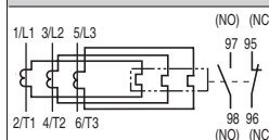
接线图
