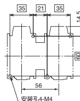
安装孔尺寸图
